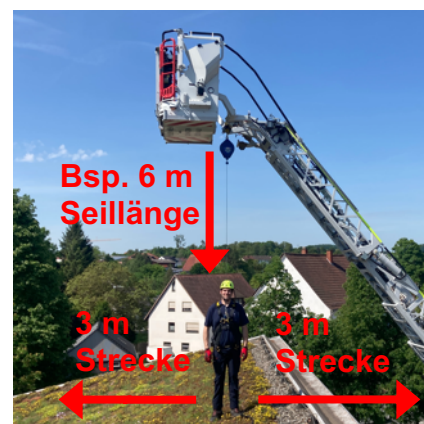
Faustformel für den Bewegungsraum wegen Winkel/ Schrägzug
