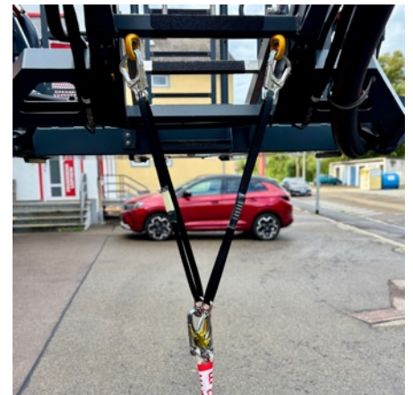
Universaladapter (seit 2025) an der Leiterspitze einer Rosenbauer Drehleiter
